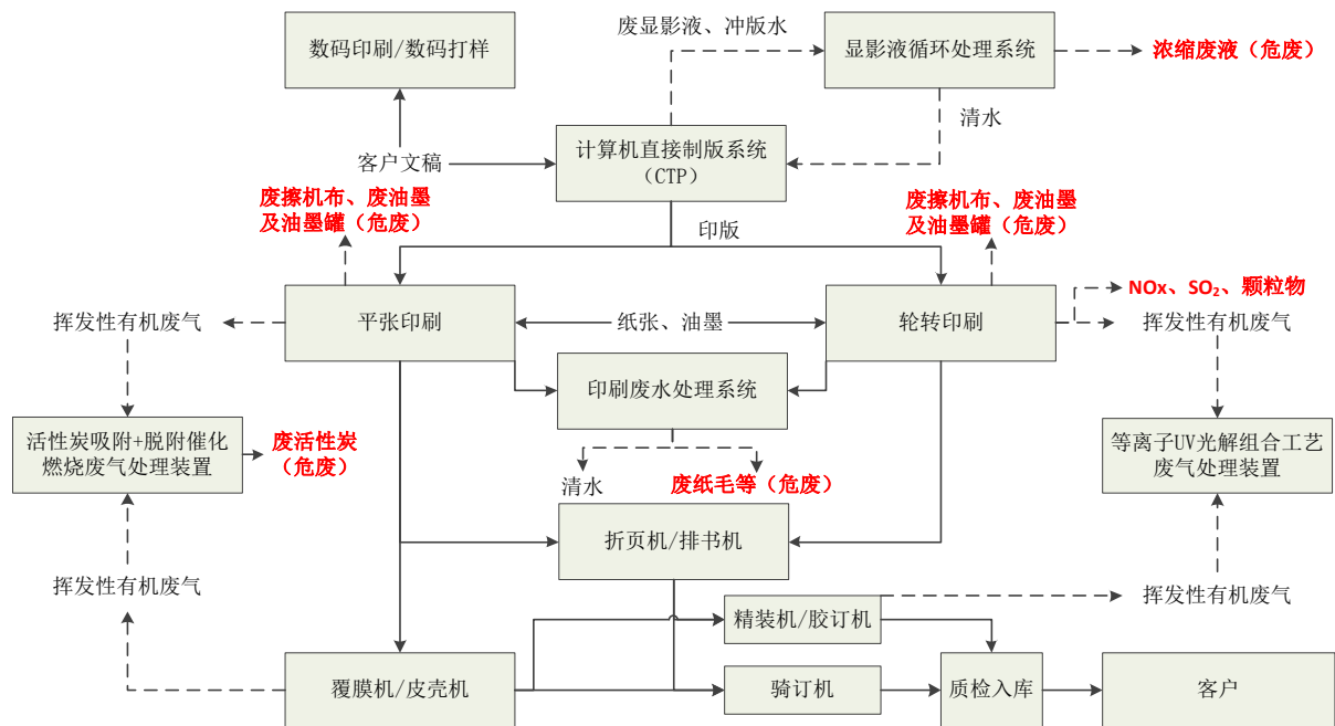
附图3 本项目生产工艺流程框图
